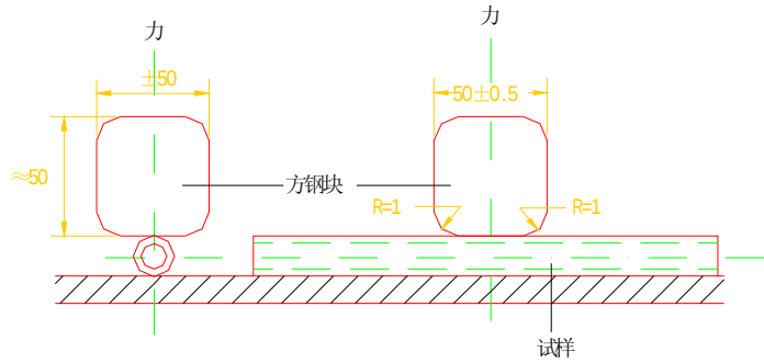
图 7 抗压试验示意图
