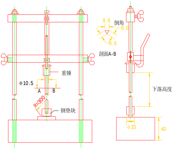
图 8 冲击试验仪
