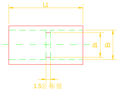
附 录 A (标准的附录) 套管配件的参照规格尺寸图
