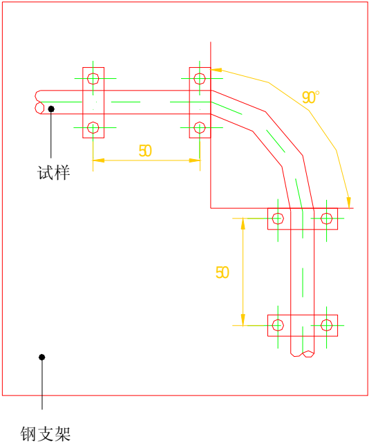
图 13 弯曲固定装置
