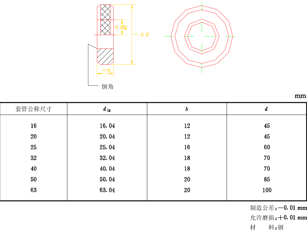
图 2 套管最大外径量规
