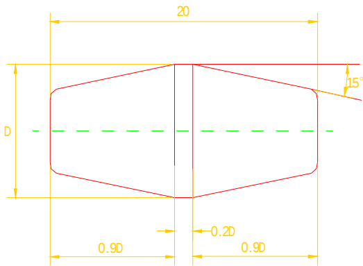
图 10 半硬质套管、波纹套管弯曲试验装置 半硬质套管及波纹套管弯曲后最小内径量规，见图 11。
