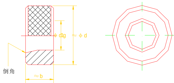
图 3 硬质套管最小外径量规 半硬质套管及波纹套管最小外径量规,见图 4。
