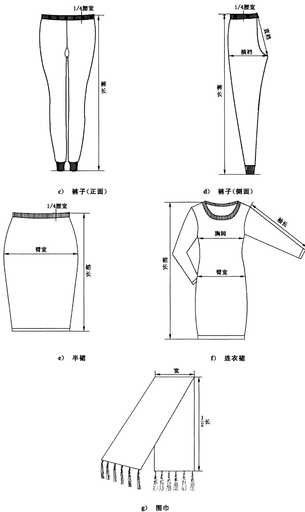
图 1 主要部位规格尺寸检验示意图(续)
