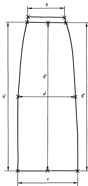
图 A.4 裙子测量部位
