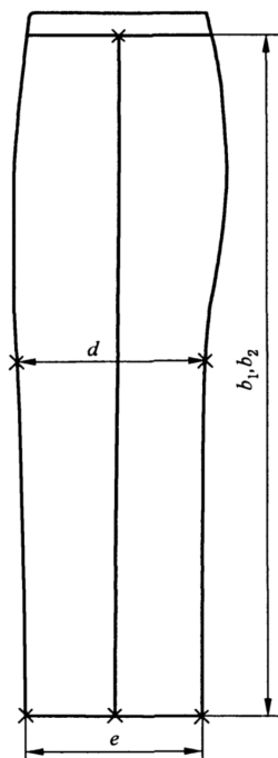
图 A.3 裤子测量部位
