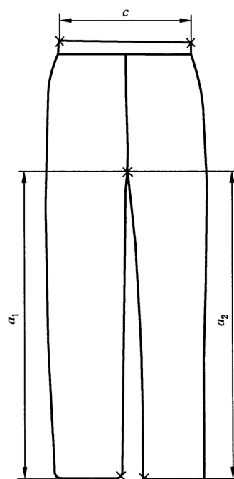
图 A.2 裤子测量部位
