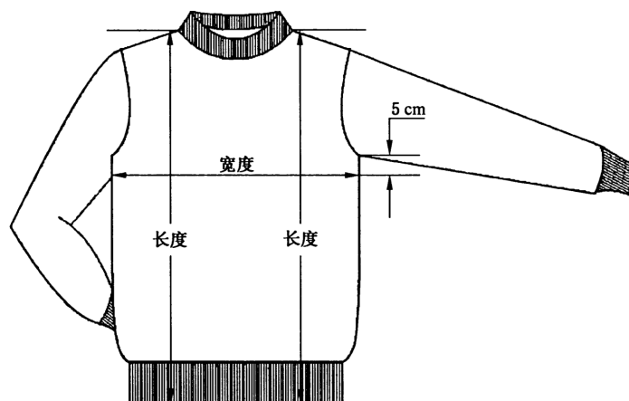
图 A.1 上衣测量部位
