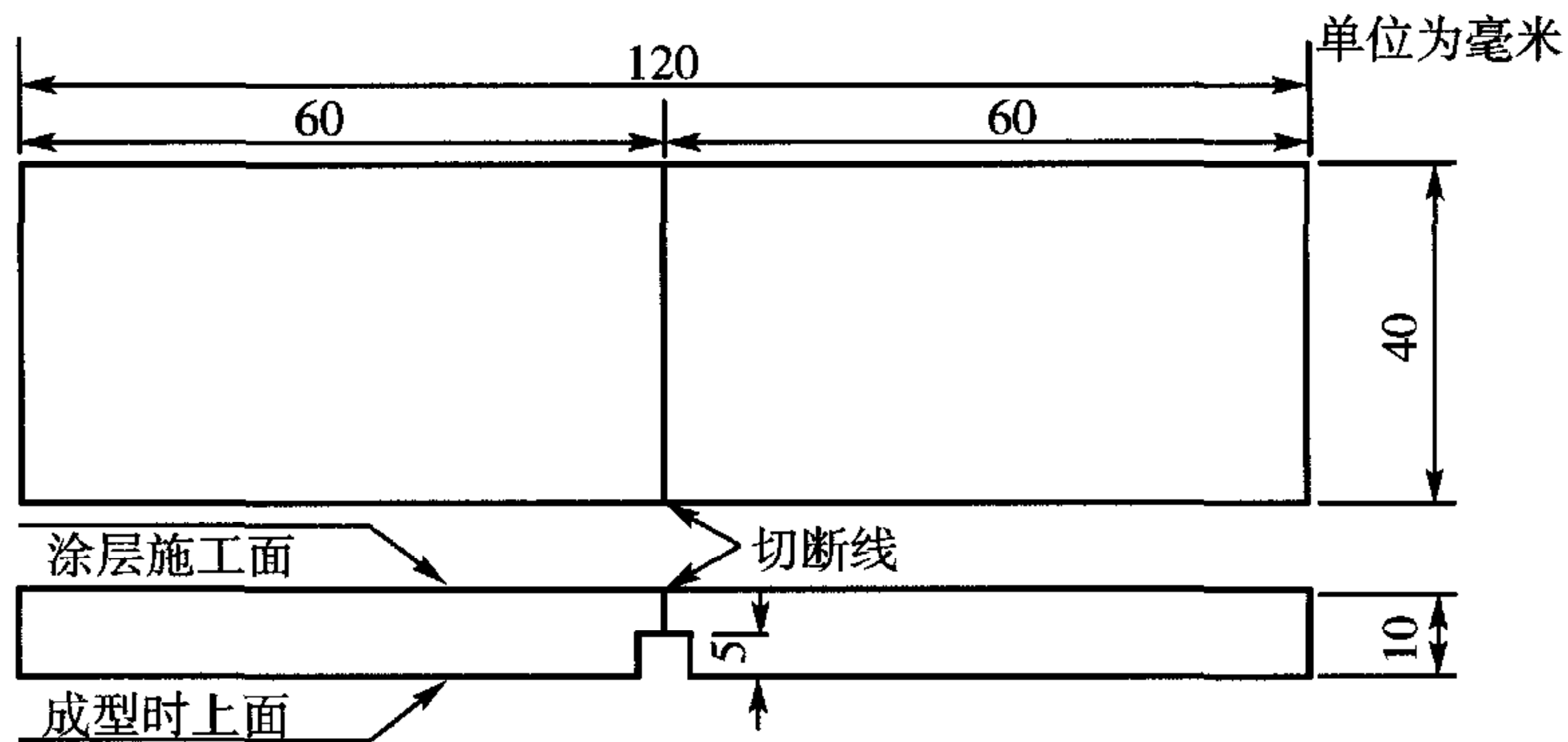
图 A.1 基材形状
