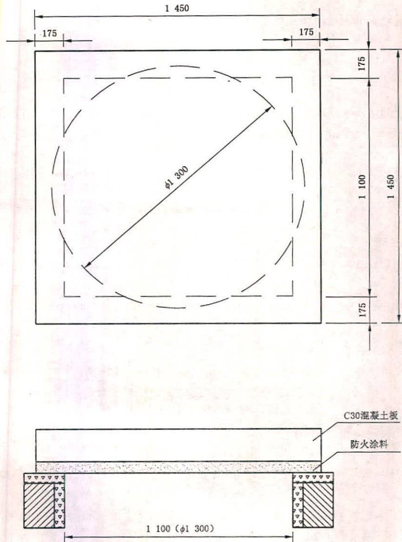
图3 耐火试件安装
