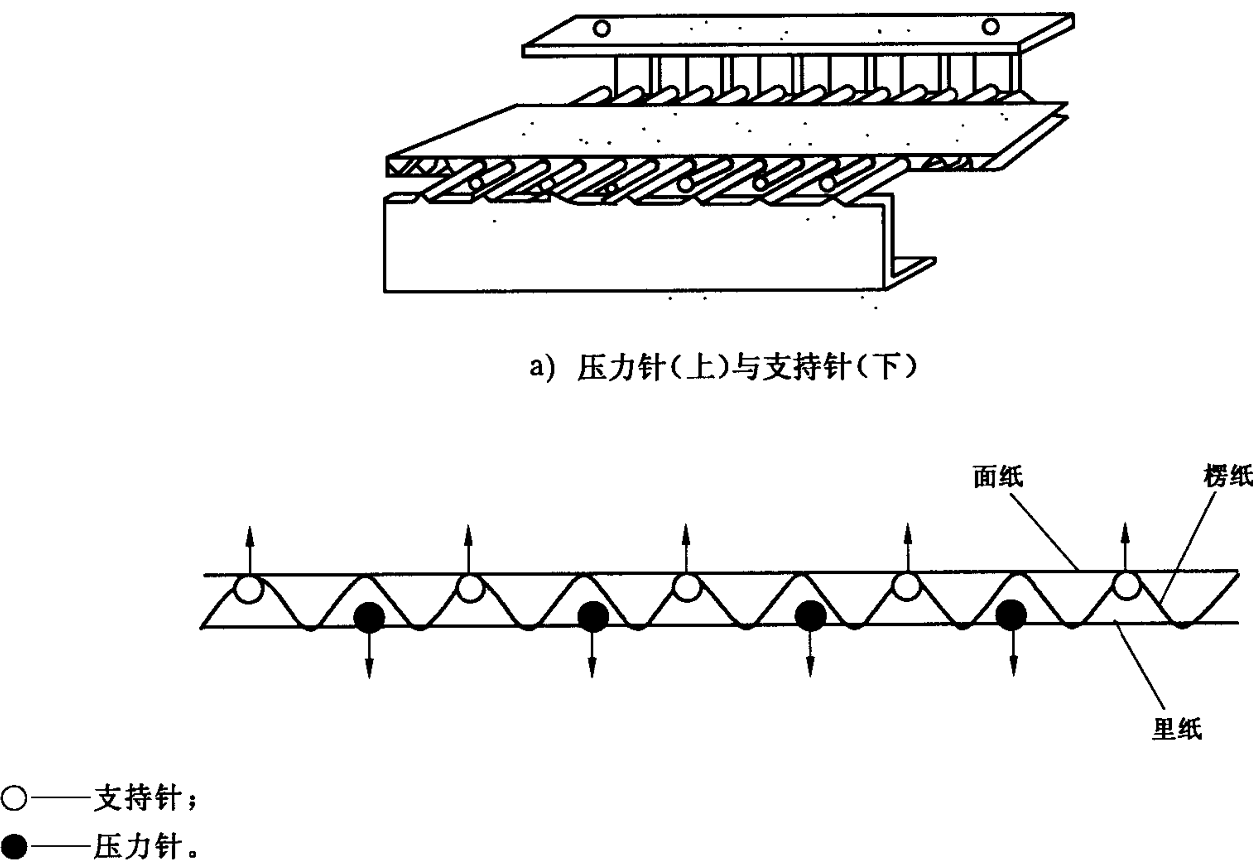
b) 压力针与支持针正面图
